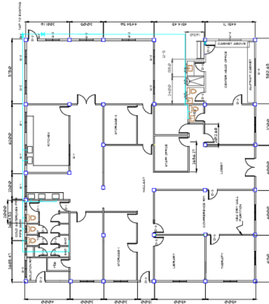
WATERLINE LAYOUT SCALE : 1 : 500
